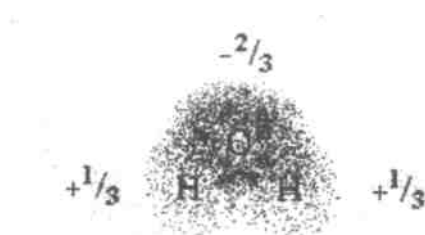
Рис. 1. Распределение заряда в атомах воды
