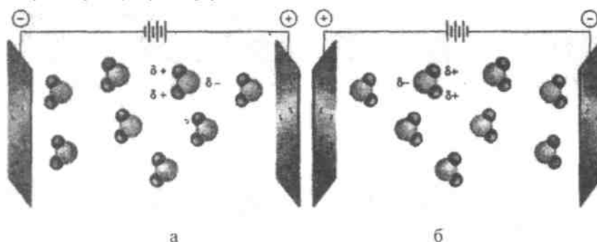
Рис. 2. Расположение молекул воды при изменении полярности напряжения
